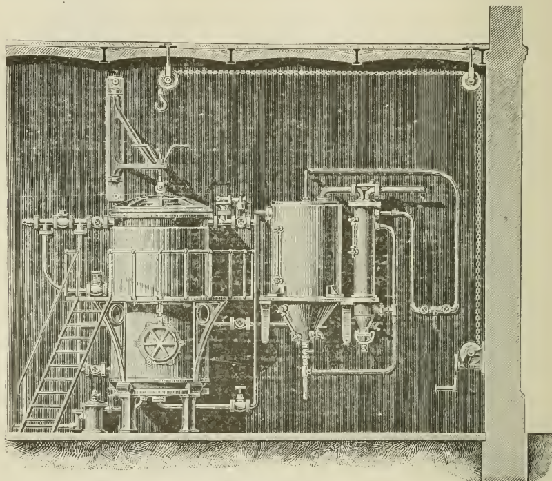
Kafill disinfectator.
